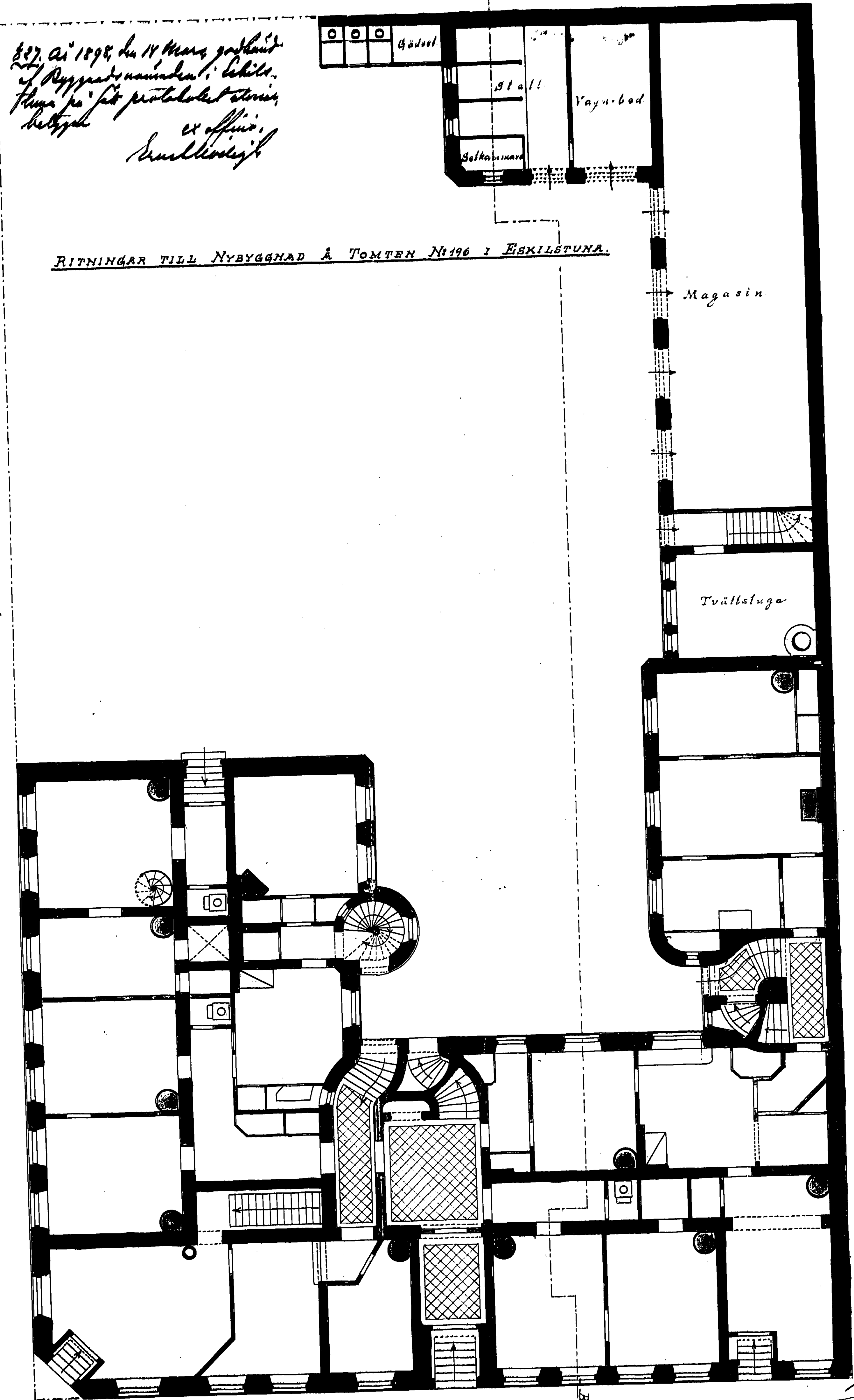
PLAN AF BOTTENVÅNINGEN
